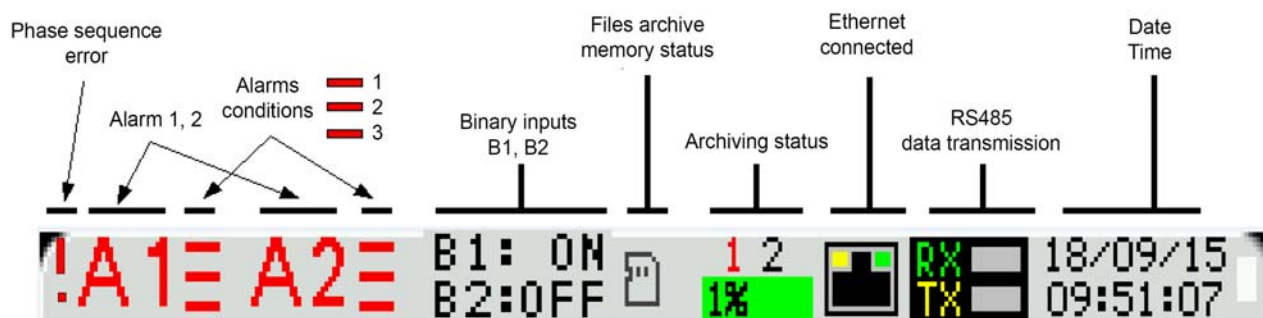
Fig. 10. Information bar
