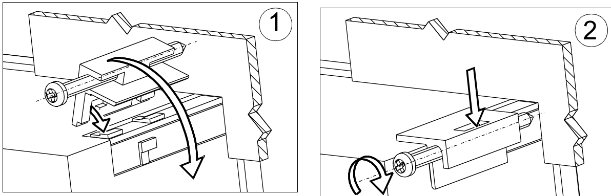
Fig. 2. Meter fitting
